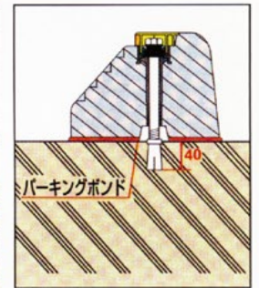
コンクリート舗装
