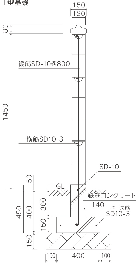
T型基礎
