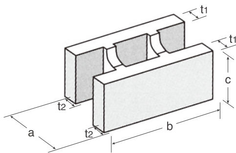
基本
