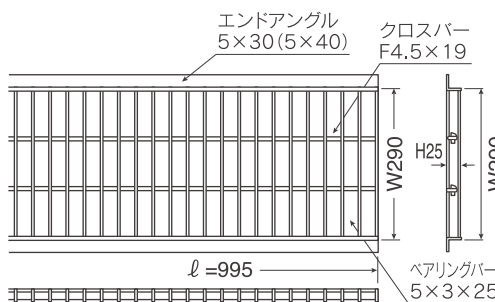
HGU-300-25L40 ( )内寸法は記号300-25L40を示す。
